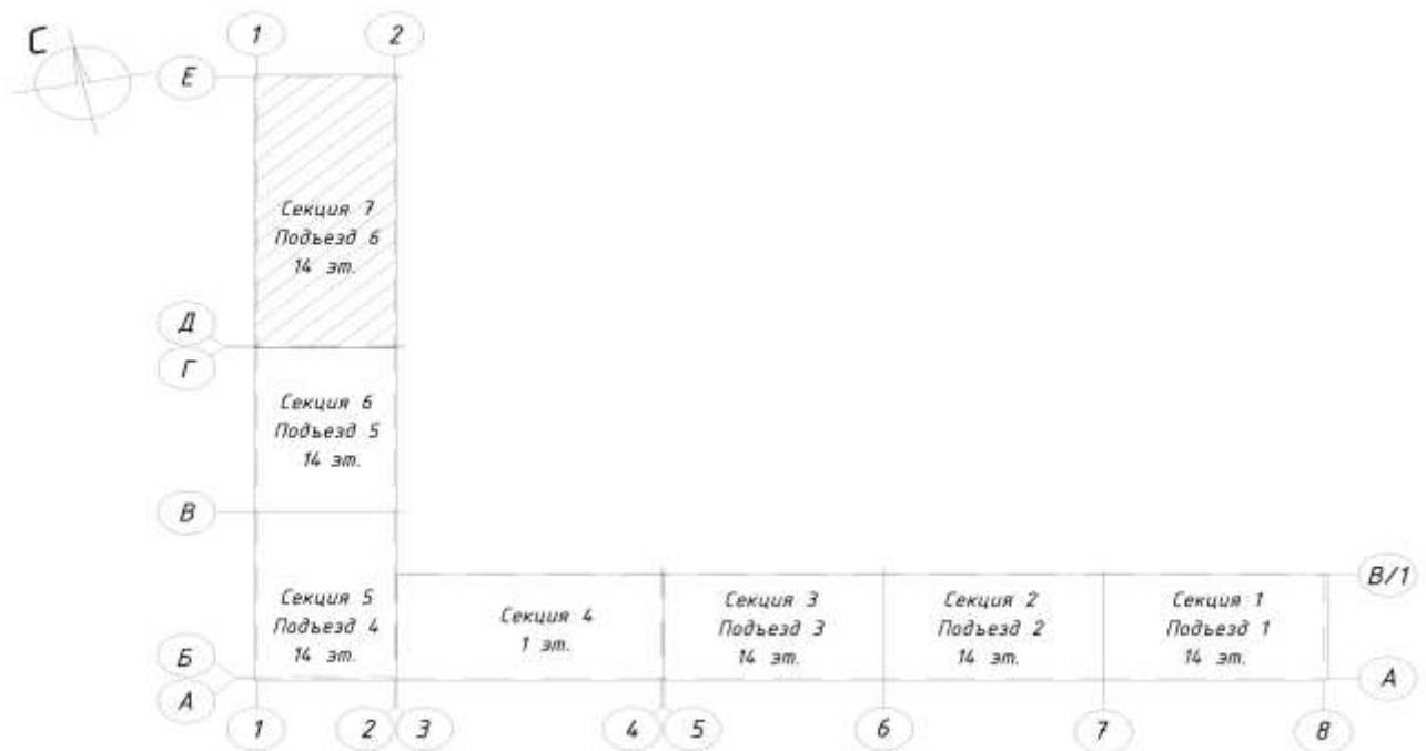
Компоновочная схема Жилой дом 15
